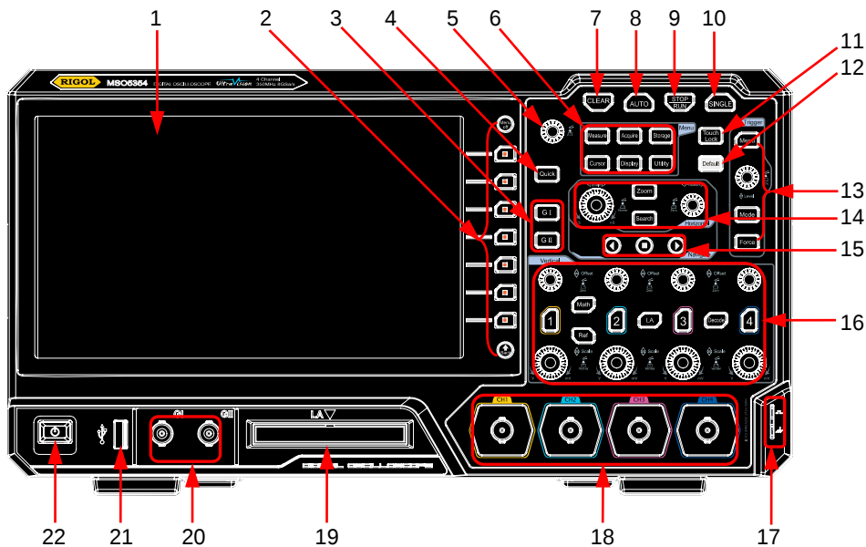
图 1-11 前面板总览
