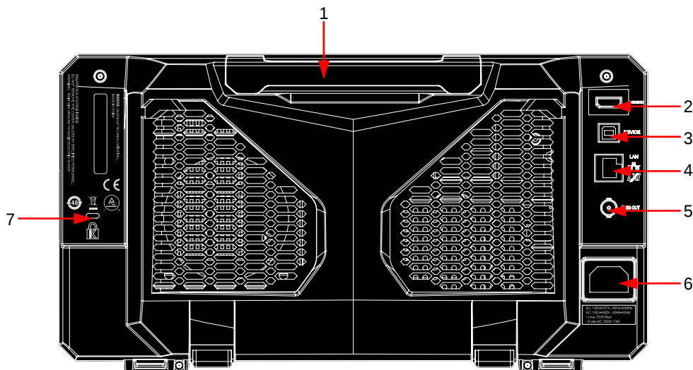
图 1-12 后面板总览
