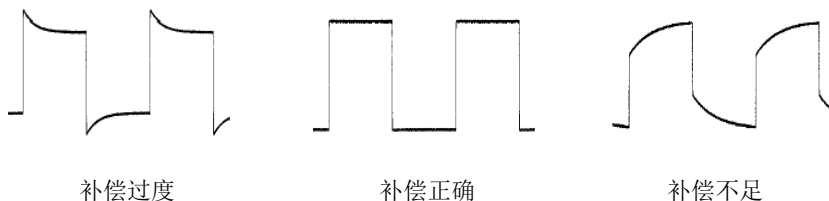
图 1-10 探头补偿
