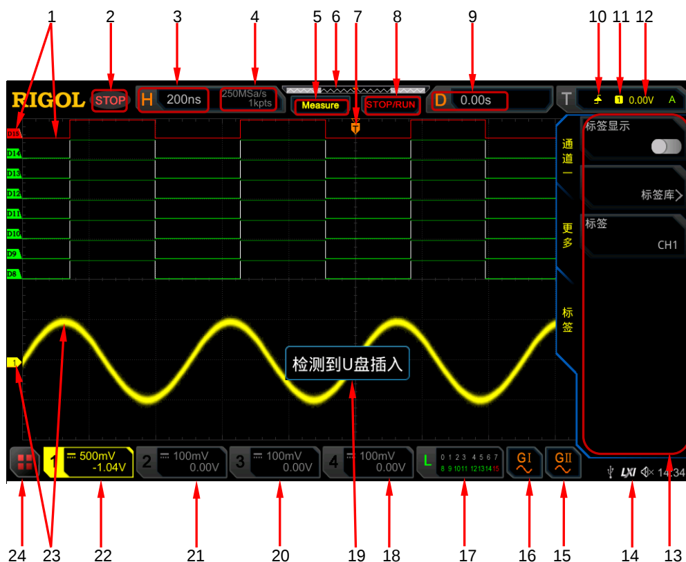
图 1-13 用户界面
